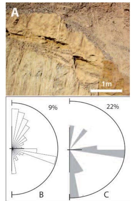
Fig. 4.- A) Falla normal. B y C) Fractura en los materiales cuaternarios y neógenos
