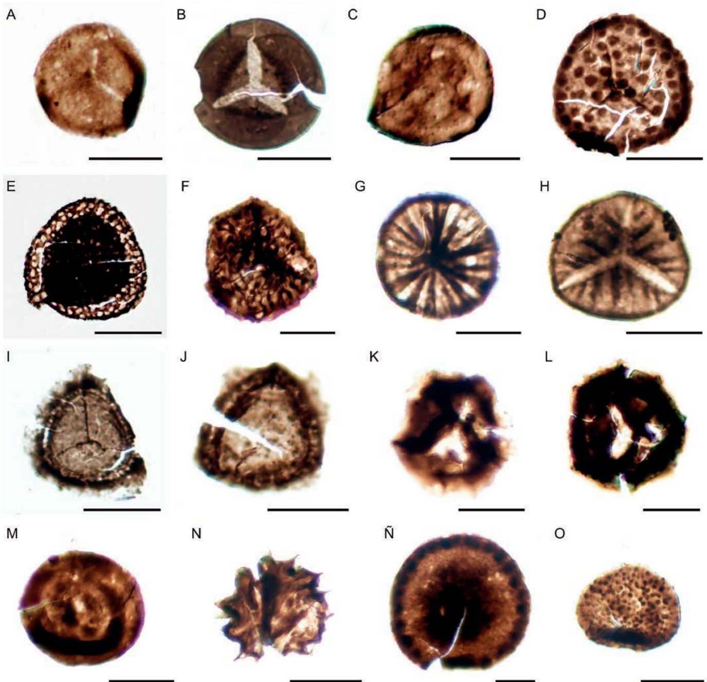
Fig. 2.- Selección de palinomorfos recuperados en la secuencia pizarroso-carbonatada al SE de Riotinto. A) Retusotriletes incohatus Sullivan 1964. B) R. rotundus Streele (Streele) 1974. C) Geminospira spongiata Higgs, Clayton y Keegan 1988. D) Epigruspora regularis González, Playford y Moreno 2005. E) Retispora lepidophyta (Kedo) Playford 1976. F) Rugospora flexuosa (Jushko) Streele 1974. G) Emphanisporites rotatus McGregor 1973. H) E. hibernicus Clayton, Higgs y Keegan 1977. I, J) Vallatisporites sp. K, L) Knoxisporites sp. cf. K. literatus (Waltz) Playford 1963. M) Tasmanites sp. N) Dupliciradiatum tenue González, Moreno y Playford 2005. Ñ) Maranhites mosesii (Brito) emend. González 2009. O) Lophosphaeridium sp. cf. L. papillatum (Staplin) Martin 1969. Barra de escala: 25 \mu m.
