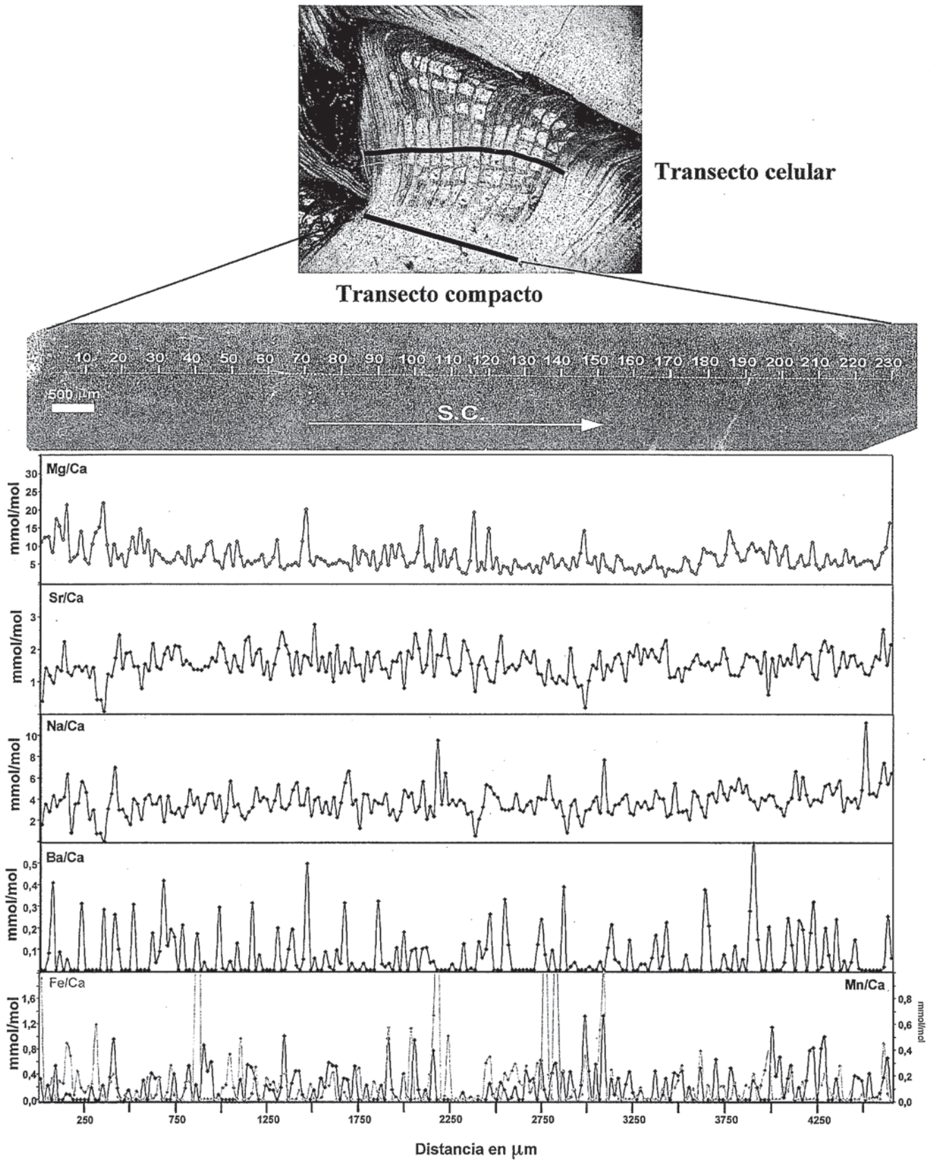
Fig.3.- Transecto a través de la microestructura compacta y distribución de las relaciones catiónicas a lo largo del mismo. S.C.: sentido de crecimiento de la concha.
