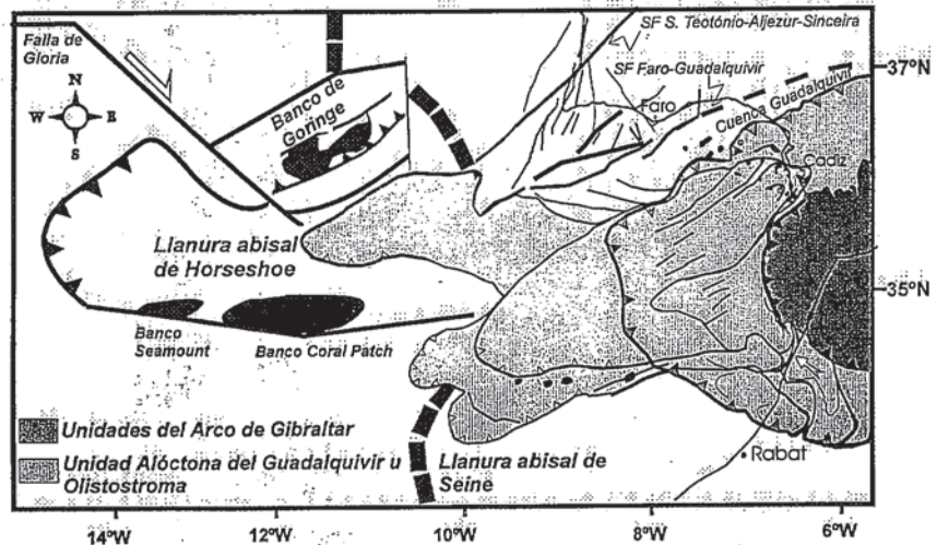
Fig. 1- Contexto tectónico del área estudiada.
