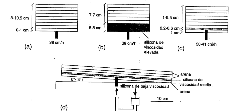
Fig. 1. Esquema del dispositivo experimental. (a) Experimentos monocapa, (b) experimentos bicapa, (c) y (d) experimentos tricapa con o sin deslizamiento gravitacional contemporáneo a la inyección.
