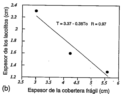
Fig. 4. Diámetro (a) y espesor (b) de los lacolitos con respecto al espesor de la cobertera de arena para la Serie-II (representada en la Fig.3). El espesor de las intrusiones ha sido representado sólo para aquellas no perforantes (modelos II-1, 2, 3, Fig. 3).
