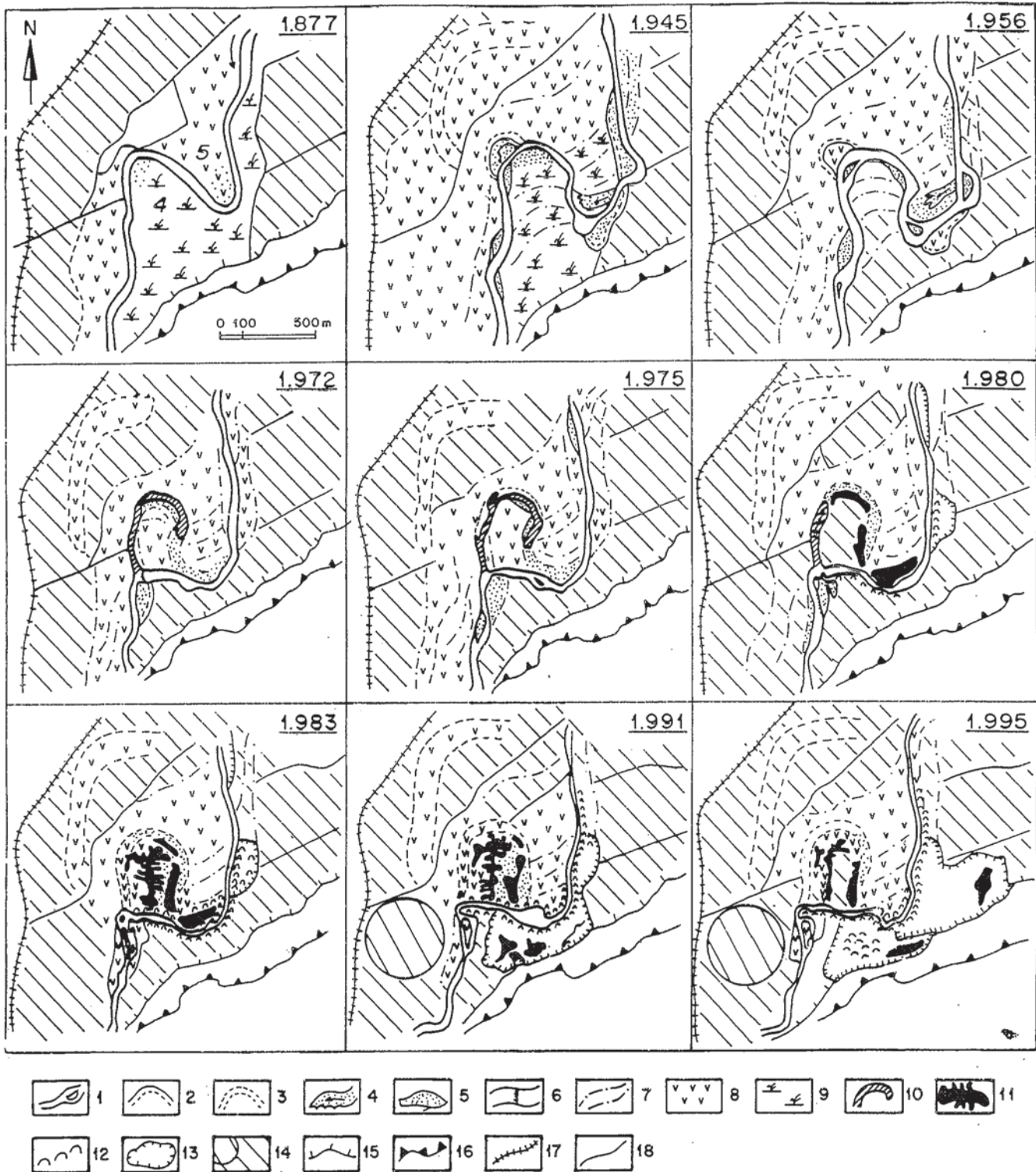
Fig.2.- Evolución de los meandros 4 y 5 del río Henares desde el año 1877 hasta 1995. Leyenda: 1) Cauce y sentido de flujo, 2) Canales secundarios de crecida, 3) Meandro abandonado, 4) Depósitos de Crevasse-splay, 5) Barras e islas, 6) Barras transversales, 7) Barras vegetadas, 8) Monte bajo, 9) Erial a pasto, 10) Laguna de yugo de buey, 11) Laguna freática, 12) Acopios y malecones artificiales, 13) Huecos mineros, 14) Cultivos, 15) Escarpe en aluviales, 16) Escarpe en yesos, 17) Ferrocarril, 18) Caminos.
