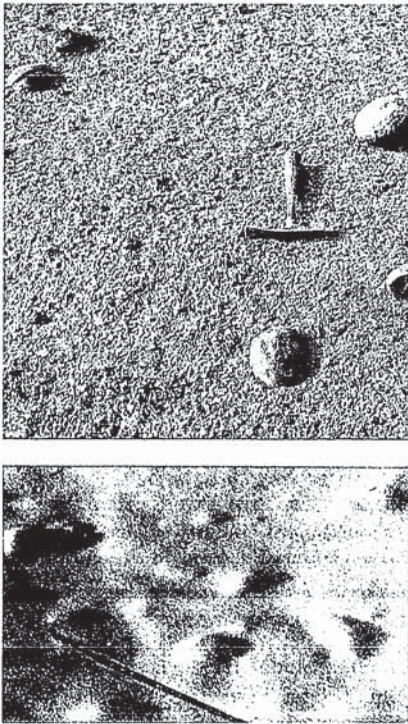
Fig. 2.- Aspecto en afloramiento de los nódulos incluidos en pizarras negras telychienses al NE de El Pobo de Dueñas (arriba), y detalle invernal del mismo (debajo), con nódulos que resaltan bajo un fino manto de nieve. Escala en dm.
