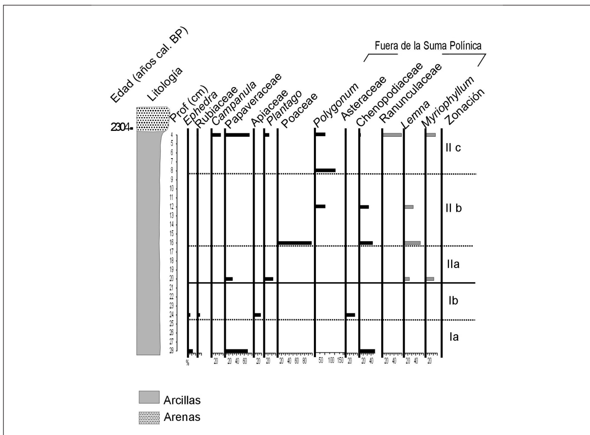
Figura 3. Vetaleña (sondeo VL-1). Diagrama polínico.
