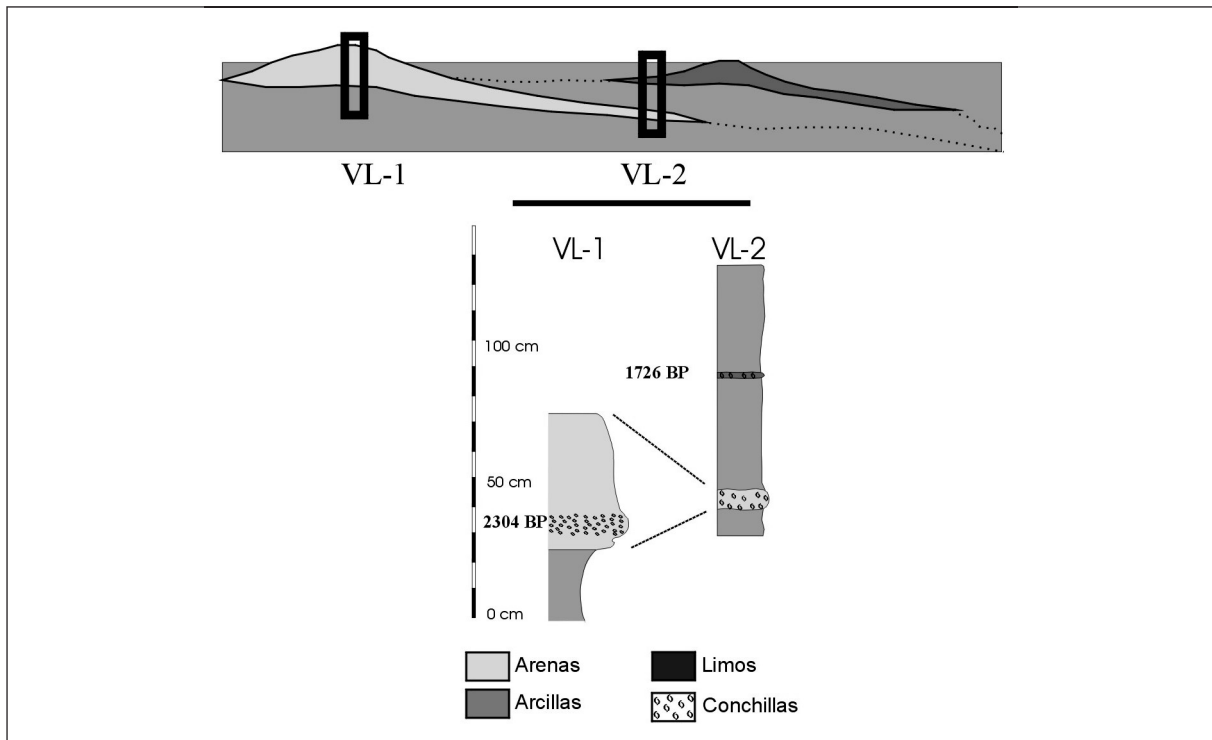
Figura 2. Litoestratigrafía y correlación de los sondeos analizados.
