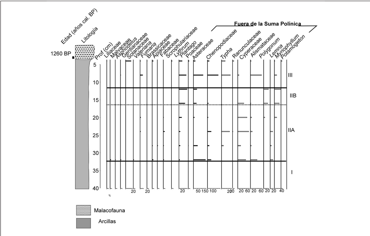
Figura 5. Vet Lengua (sondeo VL-2). Diagrama polínico.
