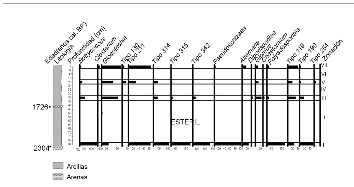
Figura 8. Vetallengua (sondeo VL-3). Diagrama de microfósiles.
