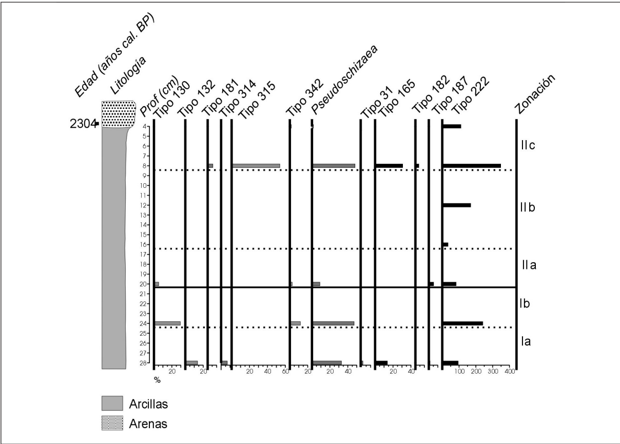
Figura 4. Vet Lengua (sondeo VL-1). Diagrama de microfósiles.
