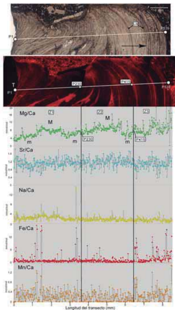
Fig. 3.- Transecto geoquímico (T) (P1-P539). Lb: Líneas b. Perfiles Mg/Ca, Sr/Ca, Na/Ca, Fe/Ca y Mn/Ca. Z1, Z2 y Z3: zonas uno, dos y tres. M: valores máximos, m: valores mínimos.
