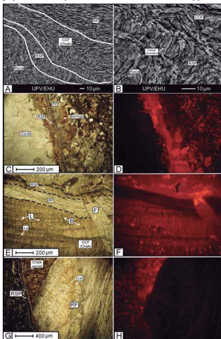
Fig. 2.- Microestructuras A) Regular simple prismática (RSP) y Regular foliada (RF). B) Detalle de A. C) RSP y RF intensamente bioturbada. D) Fotomicrografía C en catodoluminiscencia (CL). E) RSP, RF y Chalk. Situación de «blades» (B), «leaflets» (L), líneas de crecimiento b ( Lb ) y fractura F. F) Fotomicrografía E en CL. G) RSP, RF, Chalk recristalizada (Chalk recryst.) y Lb . H) Fotomicrografía G en CL.
