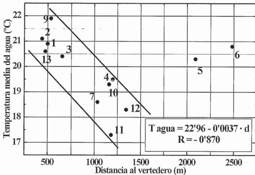
Fig. 5.- Relación entre la temperatura media del agua en los puntos de control con respecto a la distancia al vertedero de residuos sólidos urbanos de La Mina. La ecuación y el coeficiente de correlación corresponden a los 10 puntos dentro del sector indicado.
