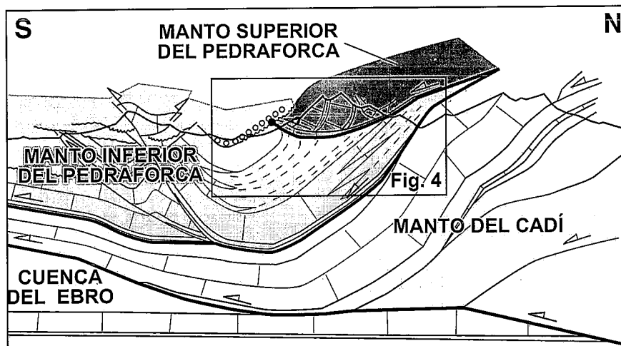
Fig. 3.- Unidades principales
