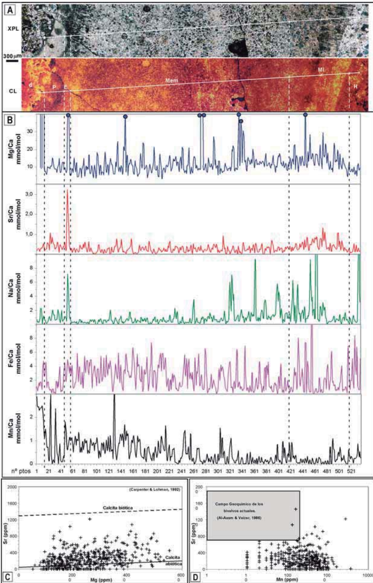
Fig. 2.- A) Transecto a través de la concha de un caprotínido (XPL, CL); dolomita (d), periostracum (P), estilolito circundánico (E) miostracum externo y medio (Mem), miostracum interno (MI), hipostracum (H). B) Relaciones catiónicas a través del transecto. C) Valores de Sr^{2+} frente a Mg^{2+} frente a la calcita biótica y abiótica. D) Valores de Sr^{2+} vs Mn^{2+} en el transecto proyectados frente al campo geoquímico de los bivalvos actuales.
