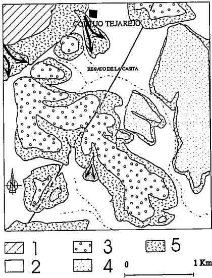
Fig. 2.- Esquema cartográfico del punto de observación del Cortijo Tejerero, al norte de la cuenca de Albarragena. 1, Cuarcitas paleozoicas. 2, Formaciones esquistograuwáquicas. 3, Raña superior. 4, Raña inferior. 5, Coluviones. FAP, Falla de Alentejo-Plasencia.
