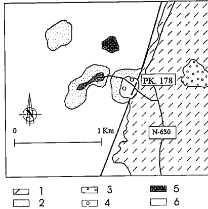
Fig. 3.- Esquema cartográfico del punto de observación en el borde oriental de la cuenca de Cañaverál. 1, Formaciones esquistograuwáquicas. 2, Sedimentos del ciclo arcóxico. 3, Terraza alta del Pleistoceno inferior. 4, Terraza de 80 m (Pleistoceno medio). 5, Terraza baja. 6, Embalse de Alcántara.
