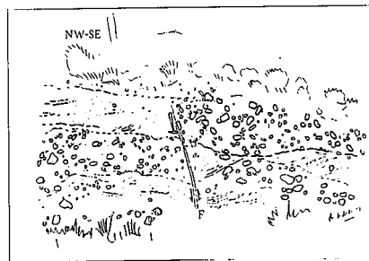
Fig. 4.- Esquema de la deformación de la terraza de 80 metros en el borde oriental de la cuenca de Cañaverál.
