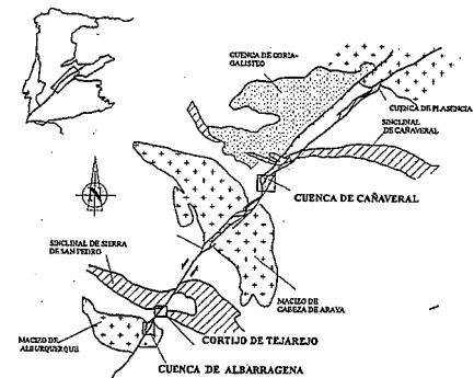
Fig. 1.- Situación de los puntos de observación descritos en la Falla de Alentejo-Plasencia.
