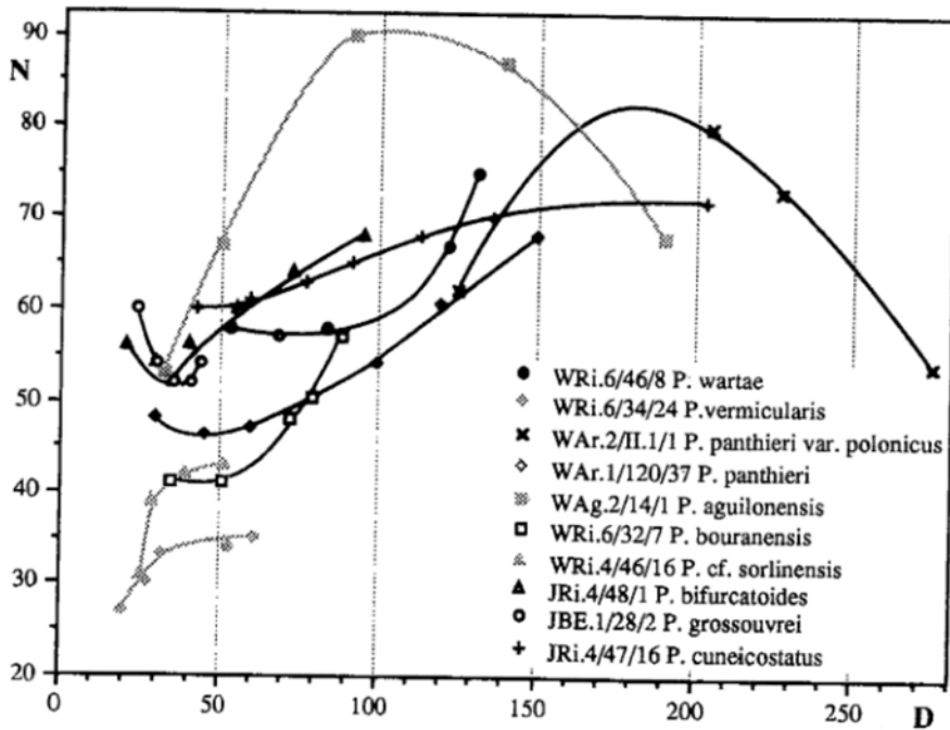
Fig 3.- Curvas de costulación de distintas formas de Perisphinctes (M y m) en el Oxfordiense Medio, (Biozonas Transversarium y Bifurcatus) de Ricla y otras localidades de la Cordillera Ibérica nororiental. Los supuestos pares dimórficos muestran una tendencia semejante en los primeros estadios. Los ejemplares de los grupos P. wartae y P. bouranensis muestran una tendencia intermedia entre las formas de la Biozona Transversarium y Bifurcatus.
