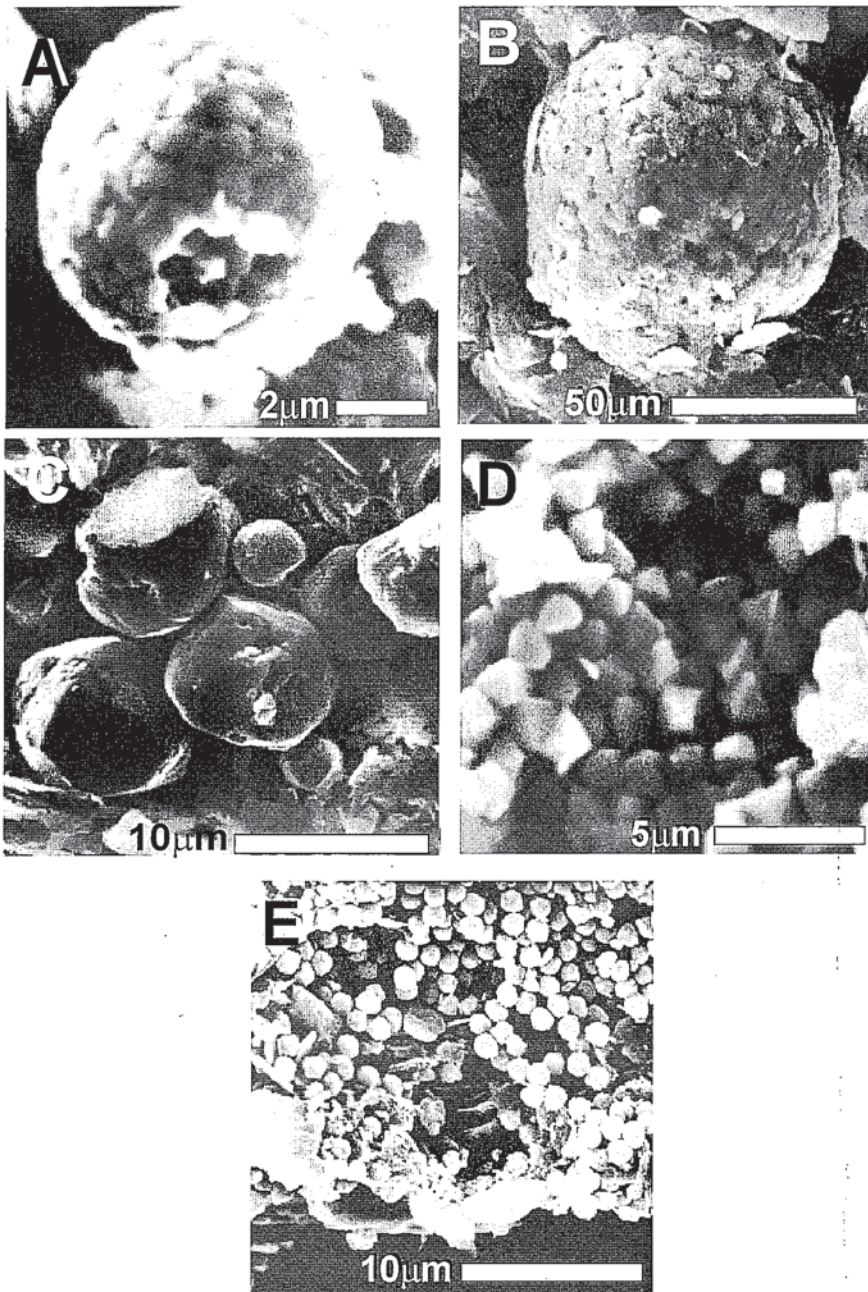
Fig. 2.- Diferentes detalles de los agregados al microscopio electrónico de barrido. A: Microframboide. B: Macroframboide. C: Macro-cristales octaédricos. D: Agregado de microcristales euhedrales. E : Agregado de microcristales subesféricos.
