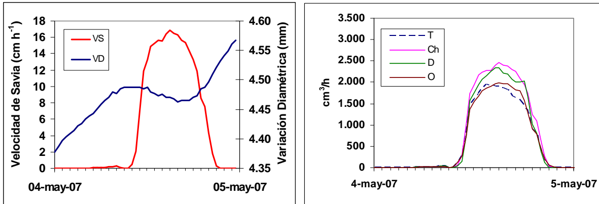
Figura 7: (izda.) Evolución diaria del diámetro del tronco y de la velocidad de la savia de Eucalyptus globulus en la provincia de Huelva. (dcha.) Evolución diaria del flujo de savia en cuatro clones de E. globulus .
