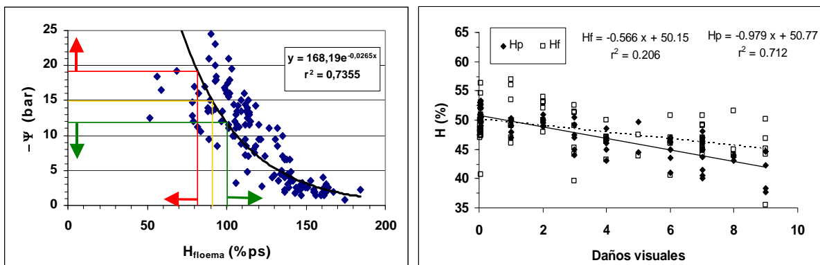
Figura 5: (izda.)Relación existente entre el contenido de humedad en floema del tronco ( H_f ), en este caso expresado respecto a peso seco, y el potencial hídrico xilemático de ramillos de la mitad de la copa ( \Psi ). El 100 y 82 % respecto a peso seco corresponden respectivamente al 50 y 45 % respecto a peso fresco. Las flechas verdes indican el rango de valores para un estado hídrico favorable, mientras que las rojas indican el rango de valores que comprometieron seriamente la supervivencia. La zona entre ambos rangos indica el intervalo de valores que causan estrés hídrico a los árboles, que cada clon soportará o no en función de su capacidad de resistencia. (dcha.) Relación entre el coeficiente de evaluación visual de daños en el tronco “Daños visuales” y el porcentaje de humedad en peridermis ( H_p : rombos, línea continua) o en floema ( H_f : cuadrados, línea punteada) (n = 75) (Fernández 2008).
