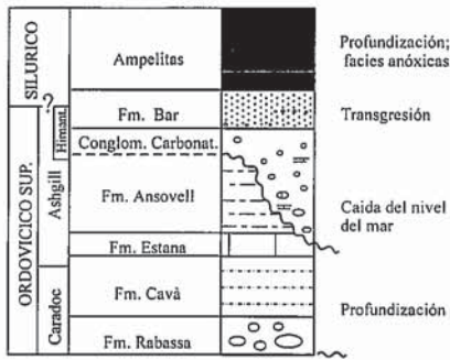
Fig. 5.- Esquema interpretativo de la sucesión del Ordovícico superior observada y su significado secuencial.
