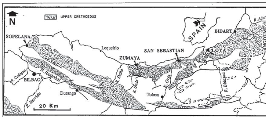
Fig. 1.- Localización geográfica de las secciones de Sopelana, Zumaya, San Sebastián, Loya y Bidart pertenecientes al Maastrichtiense medio de la Cuenca Vasca.
