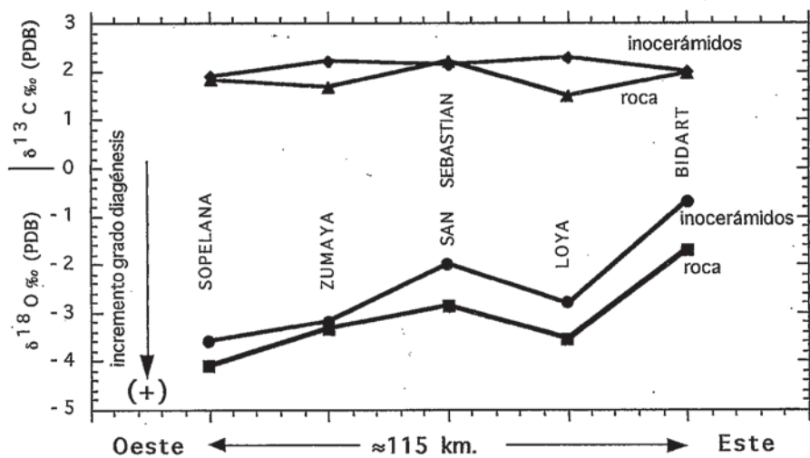
Fig. 4.- Valores medios isotópicos de carbono y oxígeno determinados en las conchas de inocerámidos y roca de las secciones So-Zu-Ss-Lo-Bi. Se aprecia una clara polaridad diagenética.
