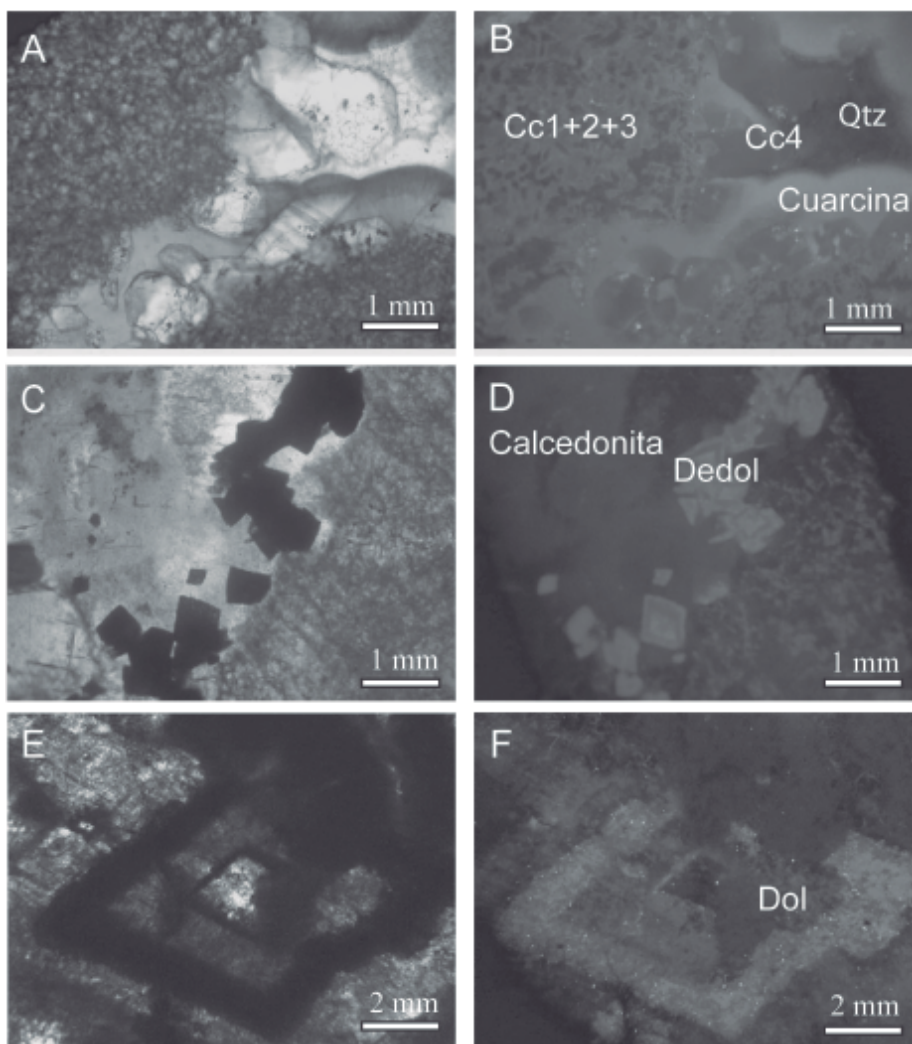
Fig. 2.- (A y B) Imagen de luz transmitida (A) y de catodoluminiscencia (B) de un coral reemplazado por Cc1, Cc2 y Cc3 y porosidad secundaria rellena de cuarzina, cuarzo y Cc4. Muestra LV-59-2. (C y D) Imagen de luz transmitida (C) y de catodoluminiscencia (D) de un nódulo de calcedonita con romboedros de dedolomita zonados en su interior. Muestra LV-A. (E y F) Imagen de luz transmitida (E) y de catodoluminiscencia (F) de un cristal zonado de dolomita tipo saddle ocupando porosidad de disolución. Muestra LV-293-2.
