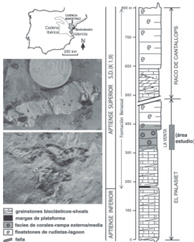
Fig. 1.- Localización, columna estratigráfica regional y fotografías de campo de las silicificaciones en las facies arrecifales.
