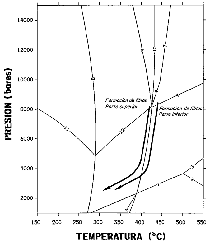
Fig. 2.- Trayectoria P-T de la formación de filitas de la Unidad de Jubrique. LISTA DE REACCIONES (las asociaciones de la izquierda son estables en la zona de temperatura superior o en la de mayor presión para las reacciones verticales)
